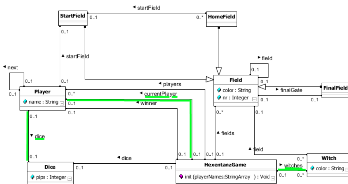
Abbildung 2: Hexentanz Klassendiagramm mit hervorgehobenen Assoziationen
