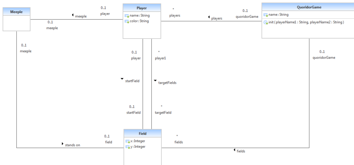
Abbildung 1: Quoridor Klassendiagramm
